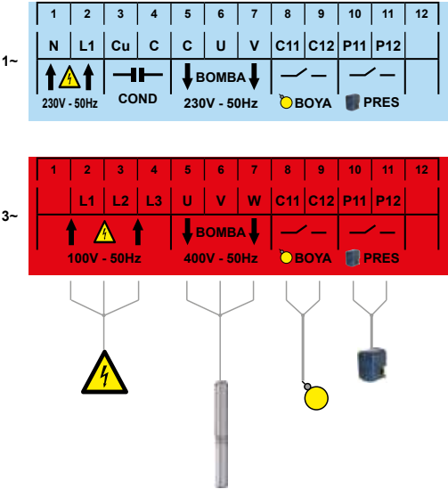
ESQUEMA DE CONEXIONES
